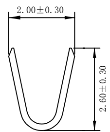
a-a SECTION
