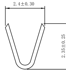
a-a SECTION
