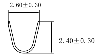
A-A SECTION
