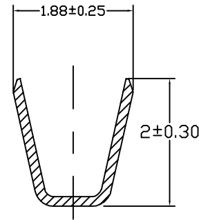
SECT.B-B
