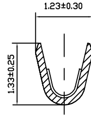
SECT.A-A
