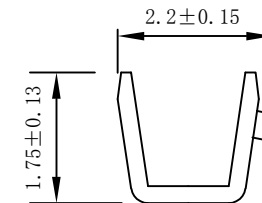
d-d SECTION
