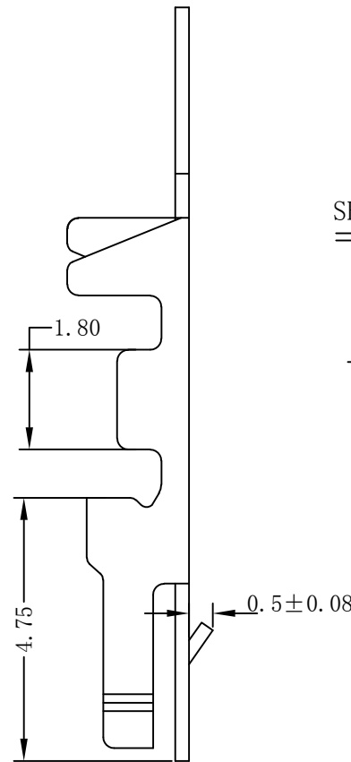
SECTION B--B
