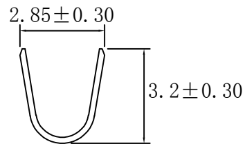
a-a SECTION
