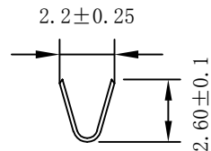
a-a SECTION
