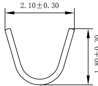
a-a SECTION
