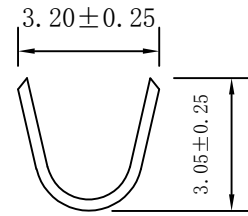
a-a SECTION
