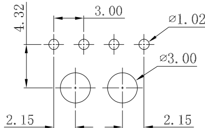
P. C. B. LAYOUT 04P-12P
