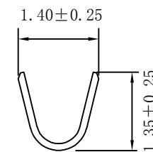
A-A SECTION
