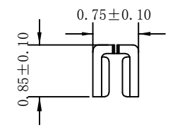
d-d section
