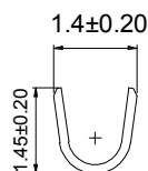
Specion B--B
