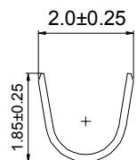
Specion A--A
