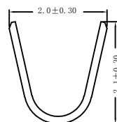
sec: a-a scale: 15/1
