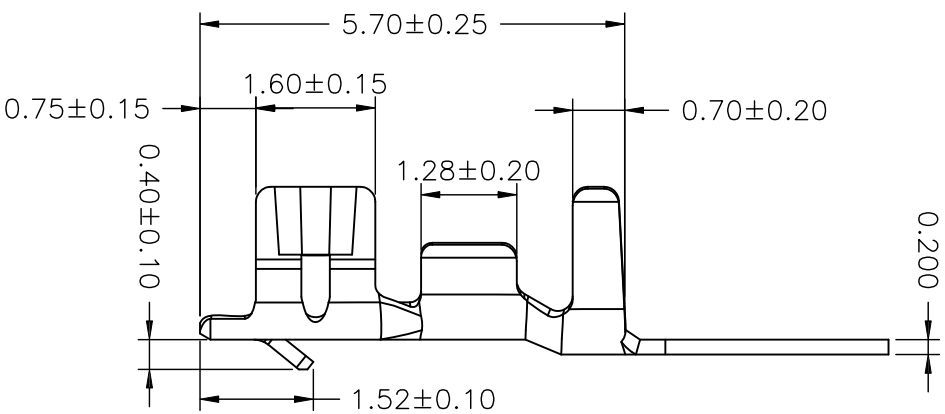
SEC:A-A
